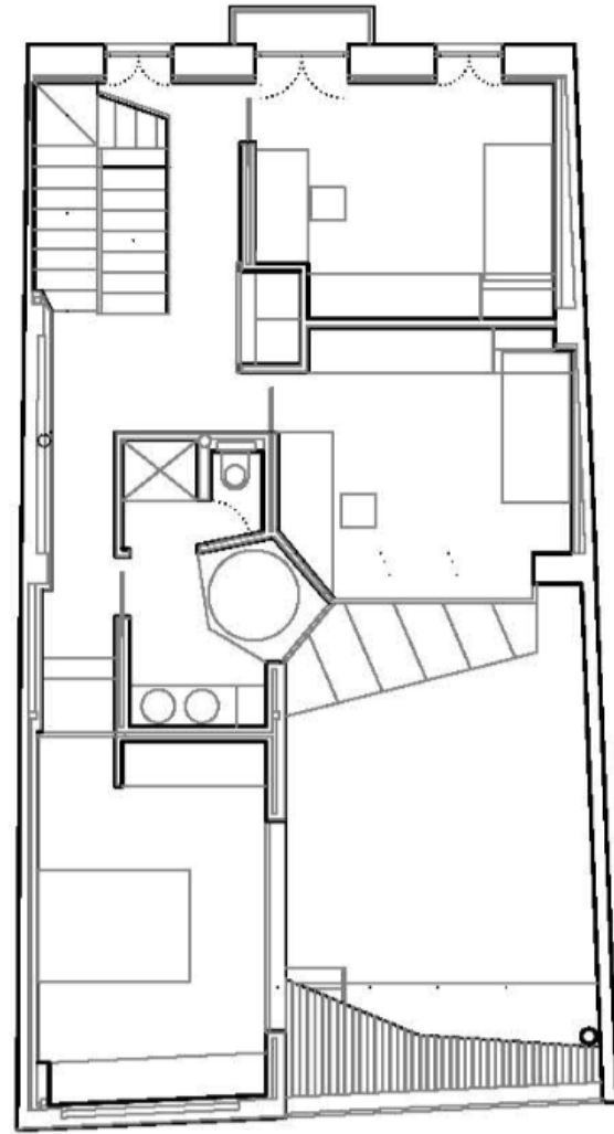
PLANTA 1
